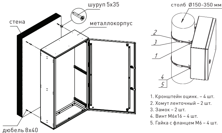
Рис. 1.1. Схема настенного монтажа.
